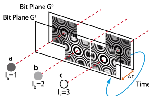
図2: 提案手法
