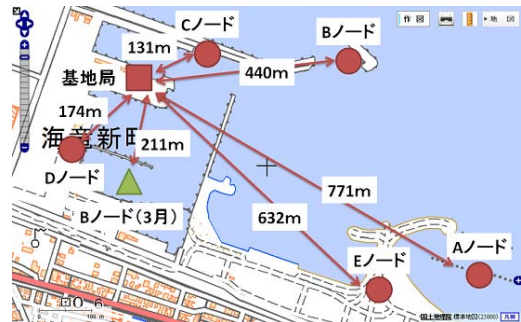
図3 観測ノードの位置関係
