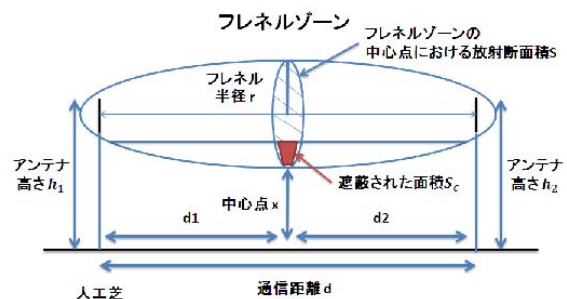
図2 フレネルゾーンの概要
