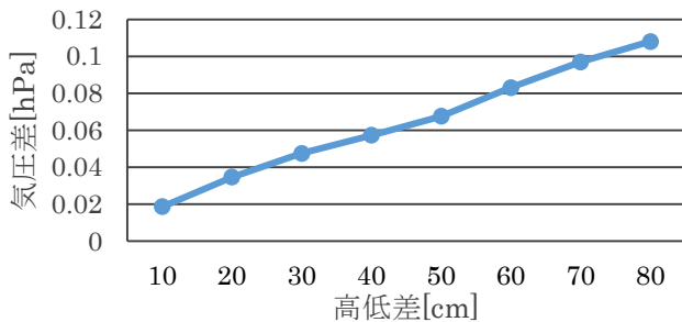
図2 高低差における気圧差
