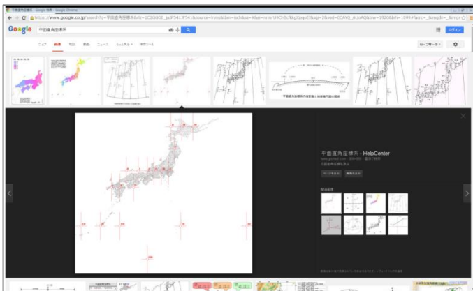
図 4 GIS の利用
