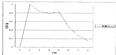
図 6.10 ロック：LPC
