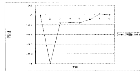
図 6.4 演歌 : LPC
