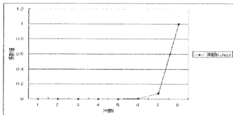
図 6.6 ジャズ：LPC
