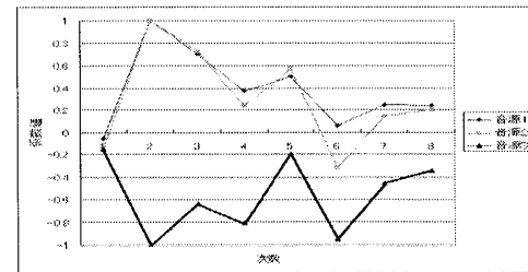
図 6.3 演歌 : 提案法
