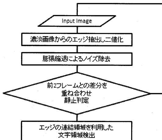
図3. 文字抽出までの処理の流れ
