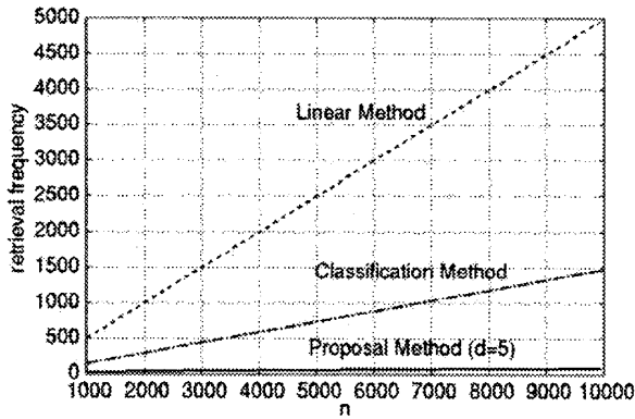
図6 平均検索回数における他の検索法との比較
