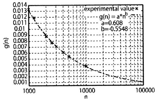
図4 照合度マトリクスサイズと検索効率
