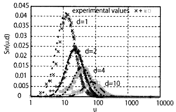
図8 検索回数分布シミュレーション
