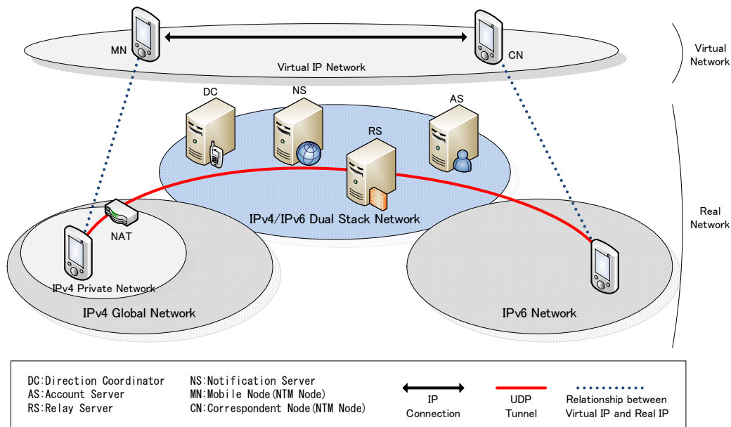
図 1 NTMobile の概要
