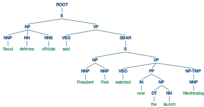
図 2 構文解析木
