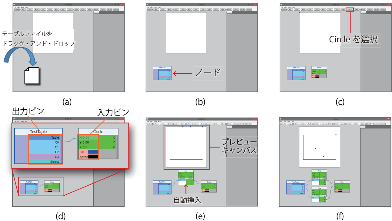
図 1 Iv Studio を用いた散布図の制作手順
