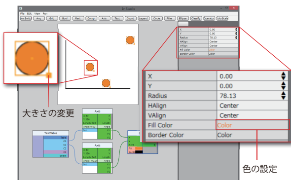
図 2 ドローツール風インターフェイスによる見た目の調整
