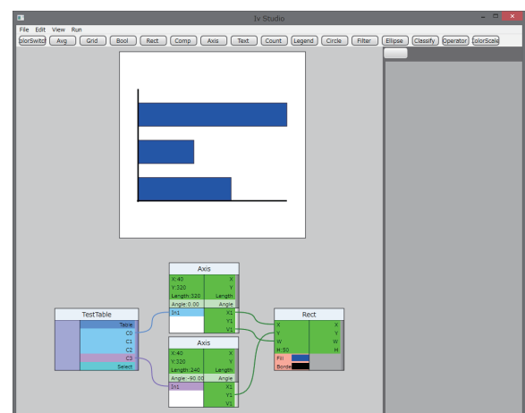
図 3 棒グラフを制作した例
