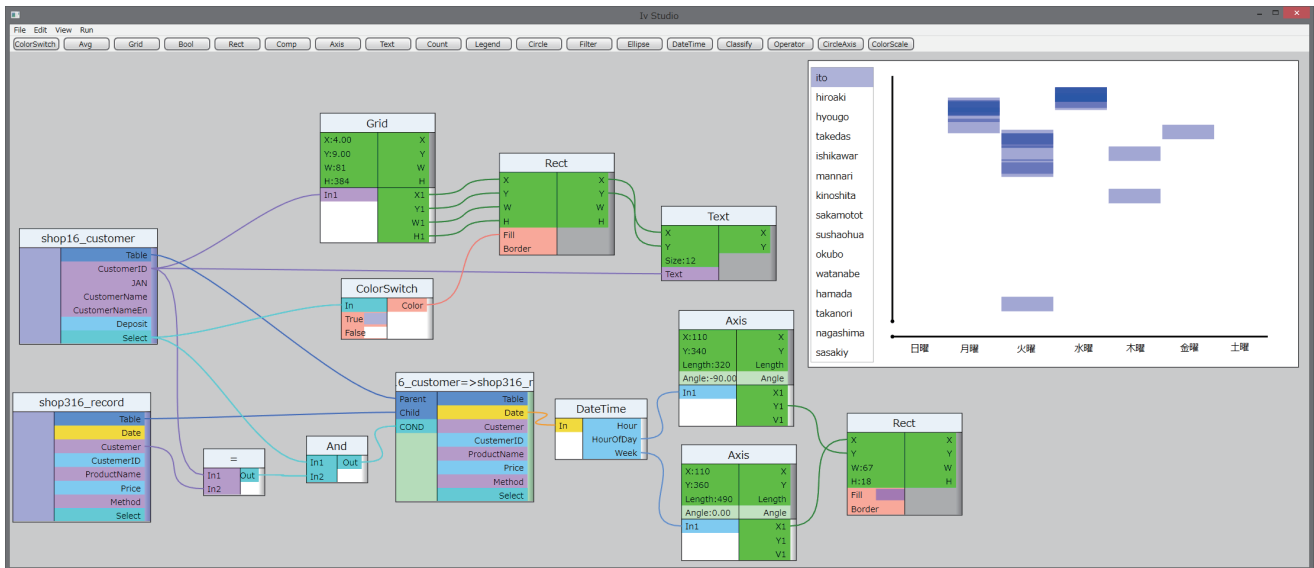
図 6 フィルタリング機能を備えた可視化手法
