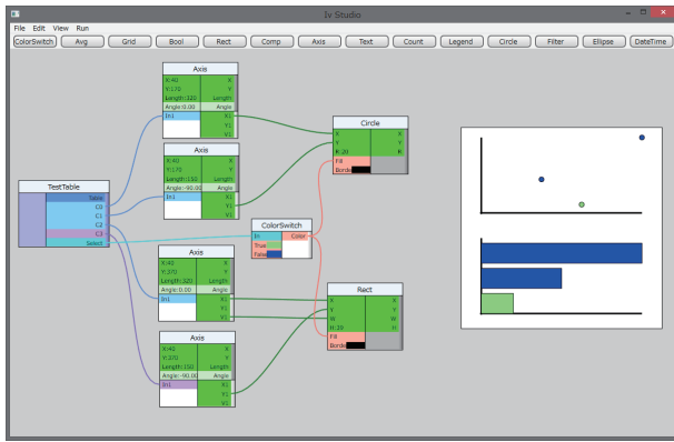
図 4 散布図と棒グラフにハイライト機能を追加した例
