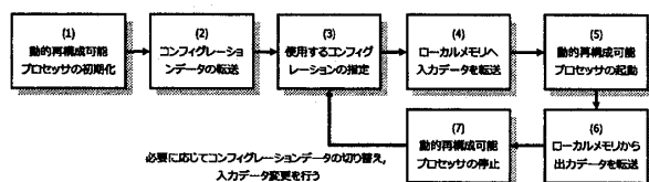
図 2: 動的再構成可能プロセッサ利用の手順
