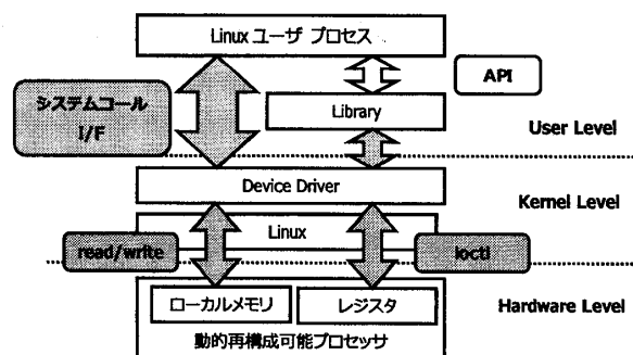
図 3: 動的再構成可能プロセッサ制御の概要
