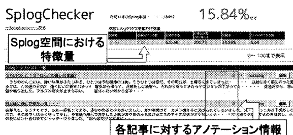
図 5: SplogChecker のユーザインタフェース
