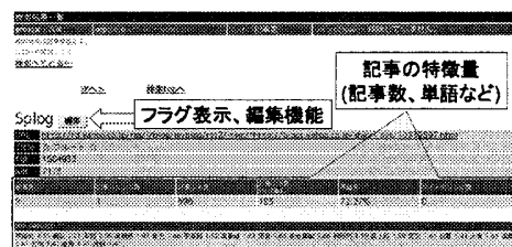
図 2: SplogAnalyzer における検索結果
