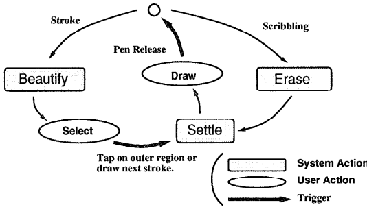
図8 対話的整形システムの動作モデル Fig. 8 Operational model of interactive beautification.
