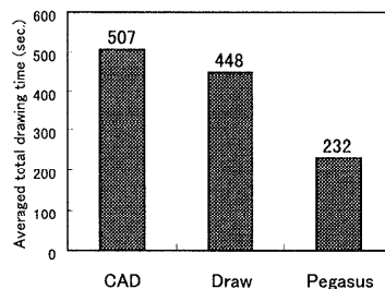
図 18 3つの図を描いた場合の推定合計描画時間 Fig. 18 Estimation for time required for a subject to draw the three diagrams.
