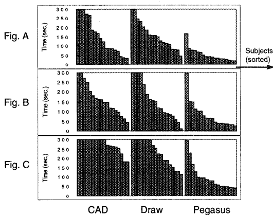
図 16 各被験者の描画時間 Fig. 16 Drawing time required for each task.
