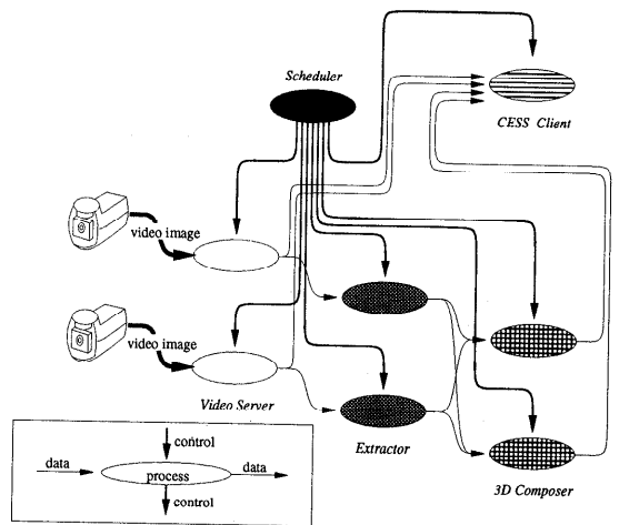
図 11 三次元再構成システムの構成
