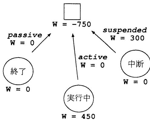
図 2: デッドロックの検出
