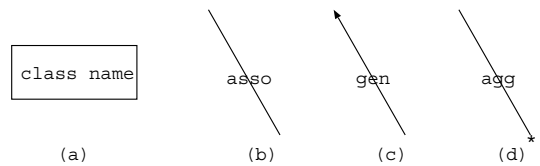
図 9 オブジェクト図の構成要素 Fig. 9 Components of the object diagrams.
