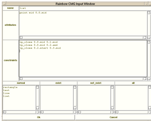
図4 「Rainbow」のCMG入力ウィンドウ(2)
