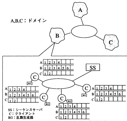
図4 拡張 ATOP のシステム構成
