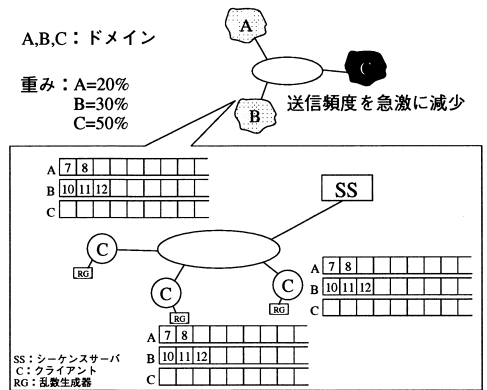
図 8 送信頻度の急激な減少
