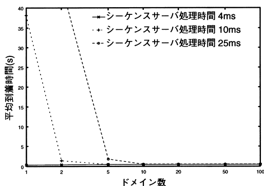
図 11 平均到着時間
