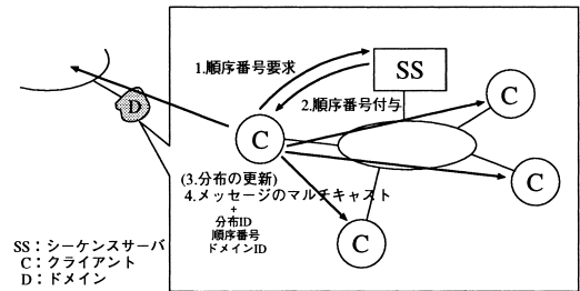
図5 メッセージの送信
