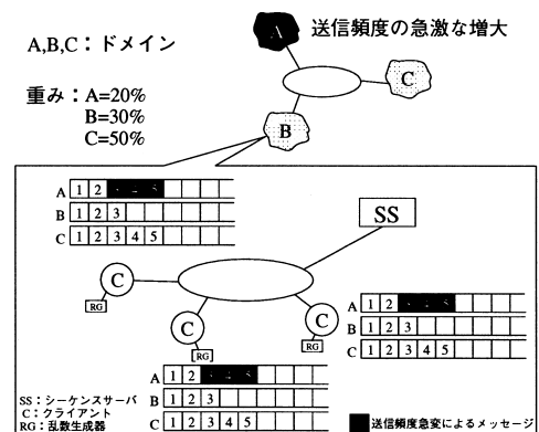
図 6 送信頻度の急激な増大
