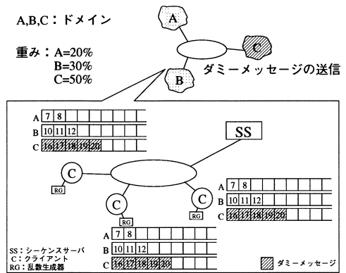
図 9 ダミーメッセージによる配送ブロックの回避
