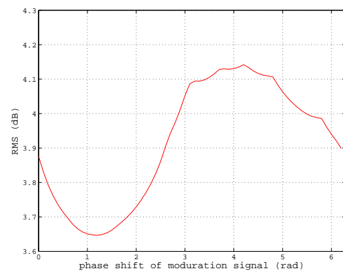
図7 モジュレーション信号の位相差 \phi と D^{(\phi)} の関係
