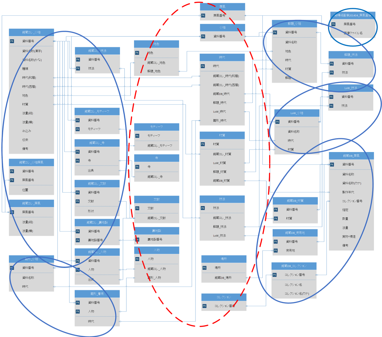
図 10 小袖屏風 DB のスキーマ Fig. 10 The scheme of Kosode Byobu Database.
