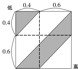
図1 不鮮明化処理における DCT 係数の変更範囲
