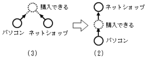
図 2 2 語の再構成
