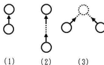
図 1 2 語の構造
