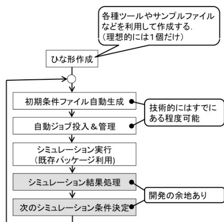
図 1 分子設計システムの概要図
