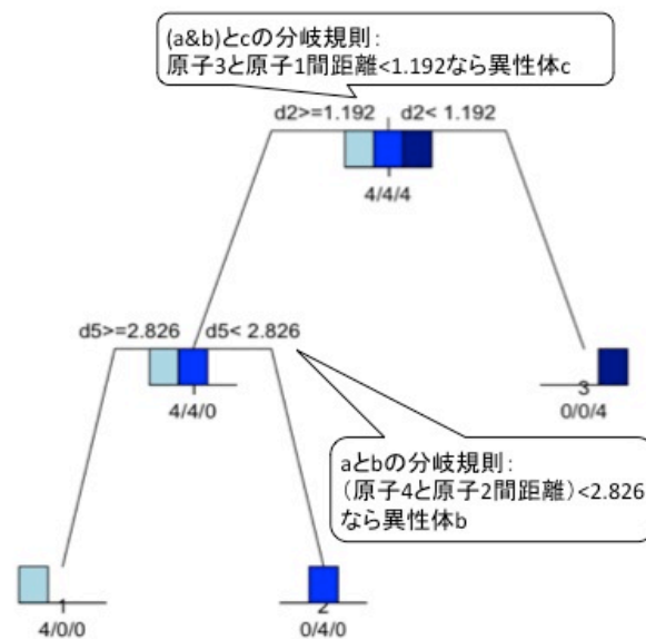
図 3 C_2H_2F_2 分子を 3 種類の異性体に分類する決定木 Figure 3 Decision tree to classify a C_2H_2F_2 molecule to 3 isomers.
