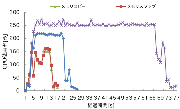
図 13 768MB 時の CPU 負荷
