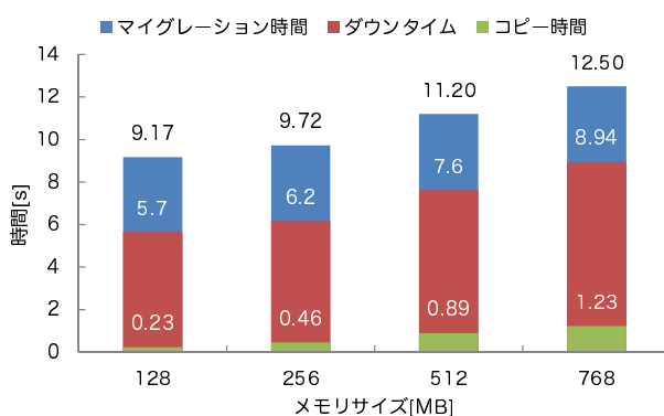
図 15 コピー・マイグレーション中のダウンタイム
