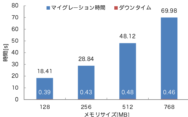
図 14 ホスト VM 間での通常のマイグレーション中のダウンタイム
