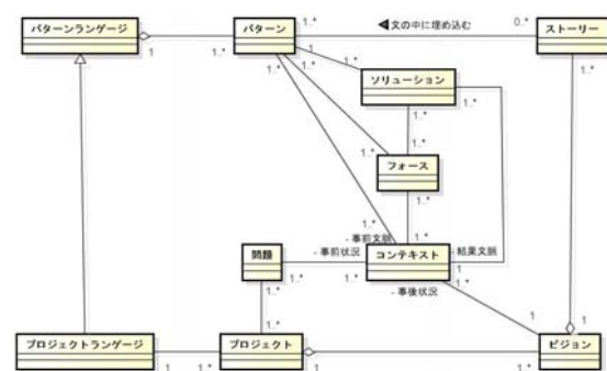
図1: パターンランゲージのメタモデル
