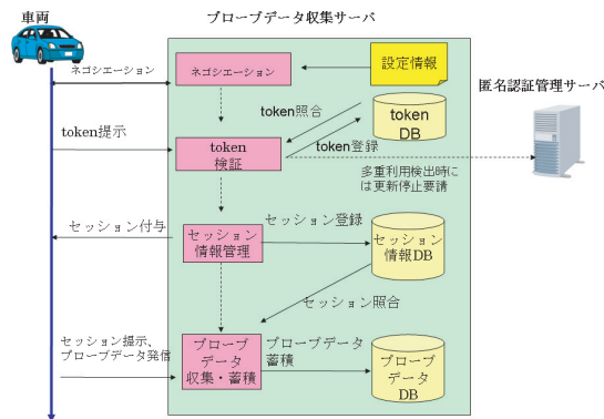
図 9 収集サーバの機能構成
