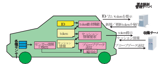
図 7 車両の機能構成
