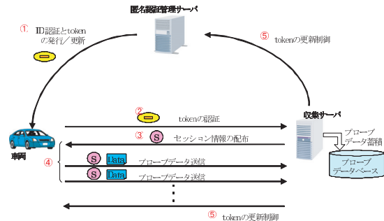
図 5 システムの構成とプローブデータの収集手順
