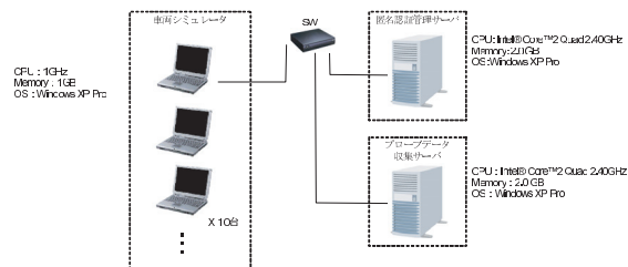
図 11 実験環境 Fig.11 Experiment environment.
