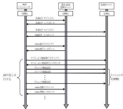
図 10 処理シーケンス Fig.10 Sequence of processes.
