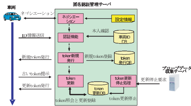
図 8 匿名認証管理サーバの機能構成
