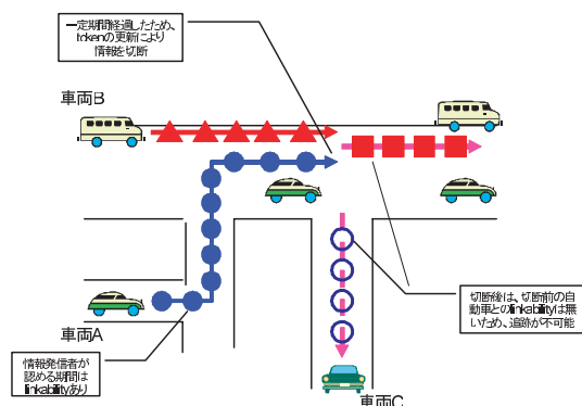
図 3 プローブ情報システムのための匿名認証方式の概念
