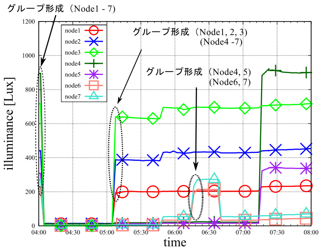
図 8 照度の変化
