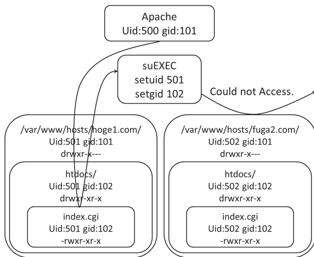
図 4 suEXEC の利用例 Fig. 4 Example for suEXEC.
