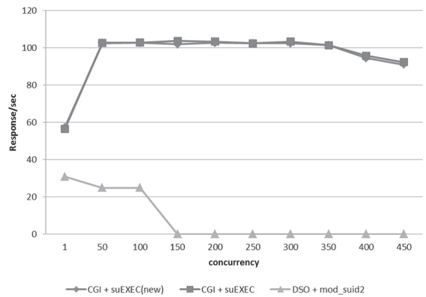
図 6 実行方式別のパフォーマンス比較
