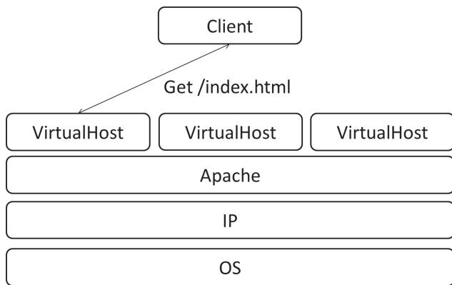
図 2 単一プロセスで複数ホストを扱う構成
