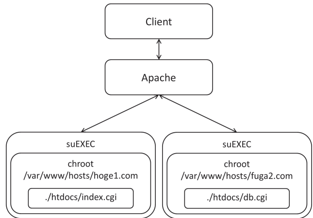
図 5 suEXEC 実行時に chroot Fig. 5 chroot on suEXEC.
