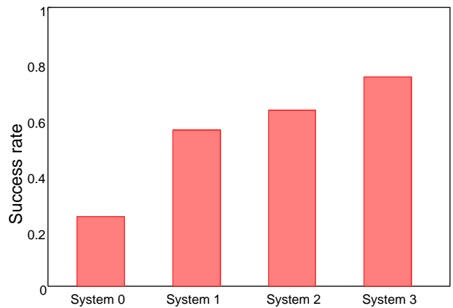
図 4 説得成功率
