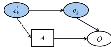
図2 ベイジアンネットワークによるベースラインモデルにおける対話状態の記述
