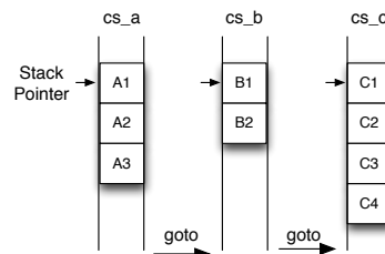
図 12 継続による引数のスタック格納の様子
