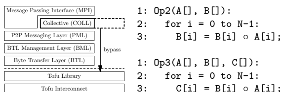
図 6 Open MPI 通信層の階層構造 図 7 演算部擬似コード
