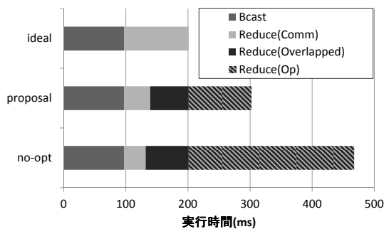
図 10 Trinaryx3 Allreduce の実行時間内訳
