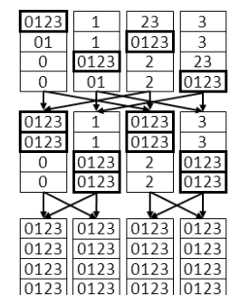
図 3 Reduce_scatter + Allgather
