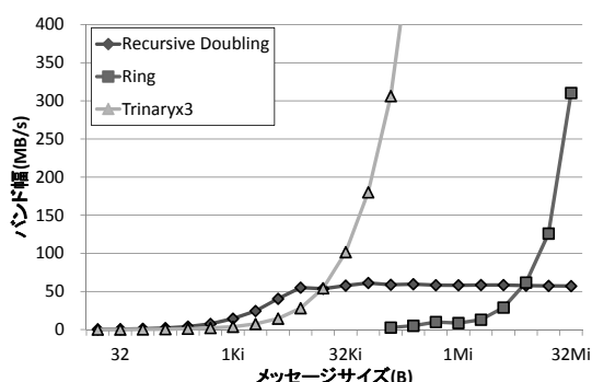
図 9 Allreduce のアルゴリズム別バンド幅 (32MiB まで)
