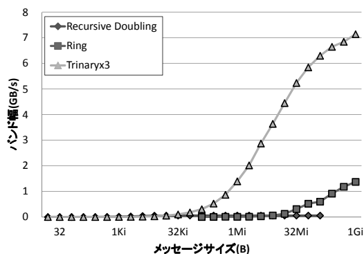
図 8 Allreduce のアルゴリズム別バンド幅 (1GiB まで)
