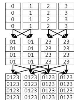
図 2 Recursive Doubling
