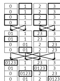
図 3 Reduce_scatter + Allgather
