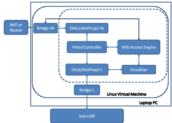
図 3 携帯型遠隔デバイス (Portable Remote Device)の構成
