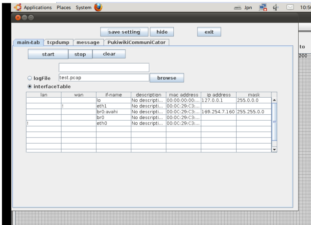
図 7 設定ウィンドウ 監視/対策インターフェース設定画面
