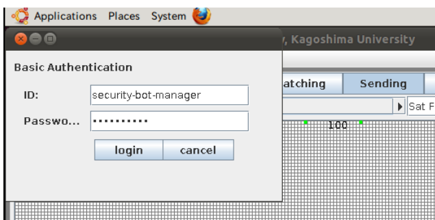
図 9 認証画面
