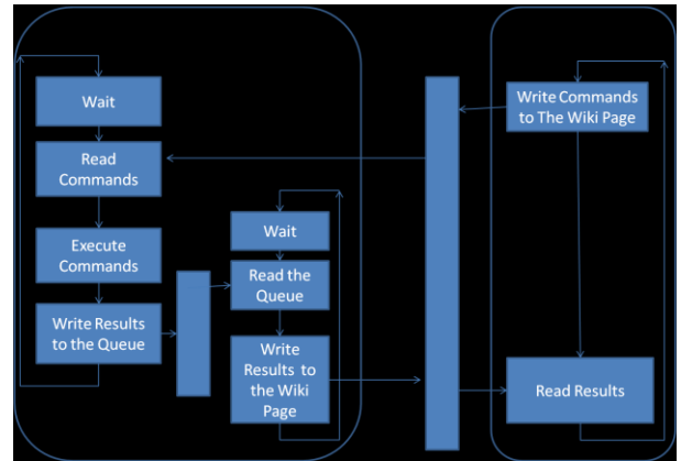
図 2 本システムの動作の概要
