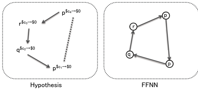
図4 ループが生じてしまうような場合の例
