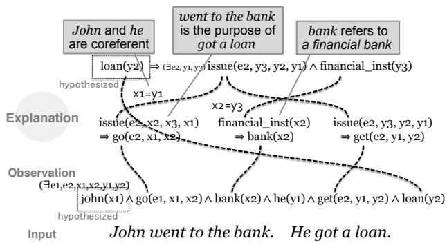
図1 仮説推論による言語理解の例
