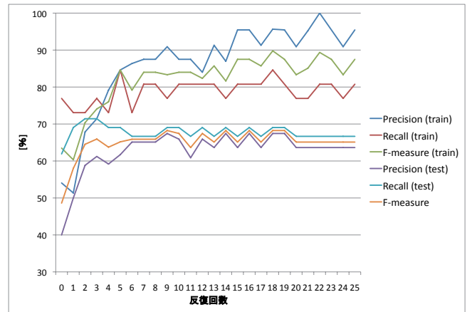
図5 反復回数ごとの実験結果
