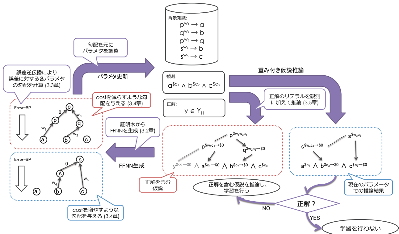
図2 提案手法の概要
