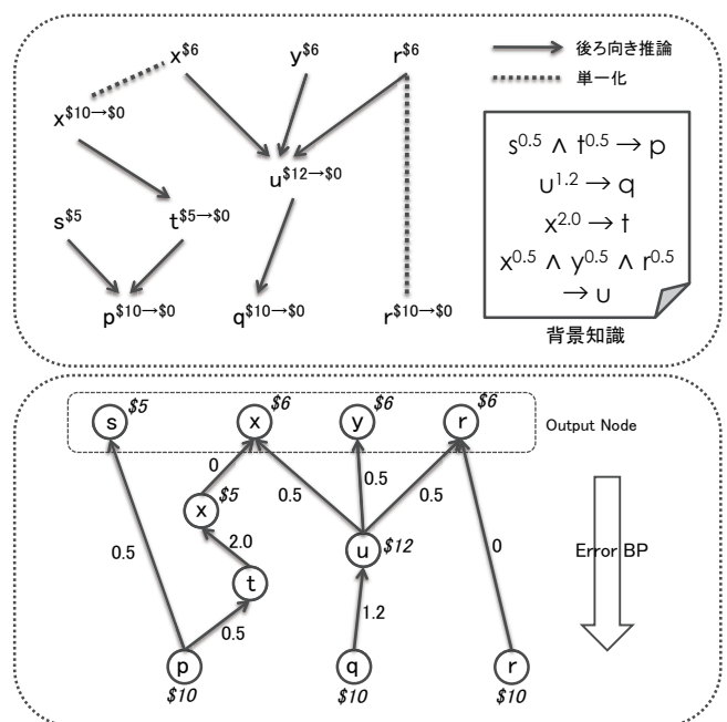
図3 推論グラフから FFNN への変換例
