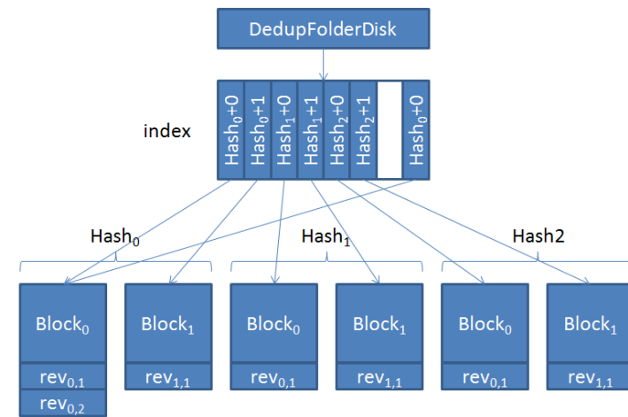
図 2. DedupFolderDisk の構造 Fig.2 The structure of DedupFolderDisk
