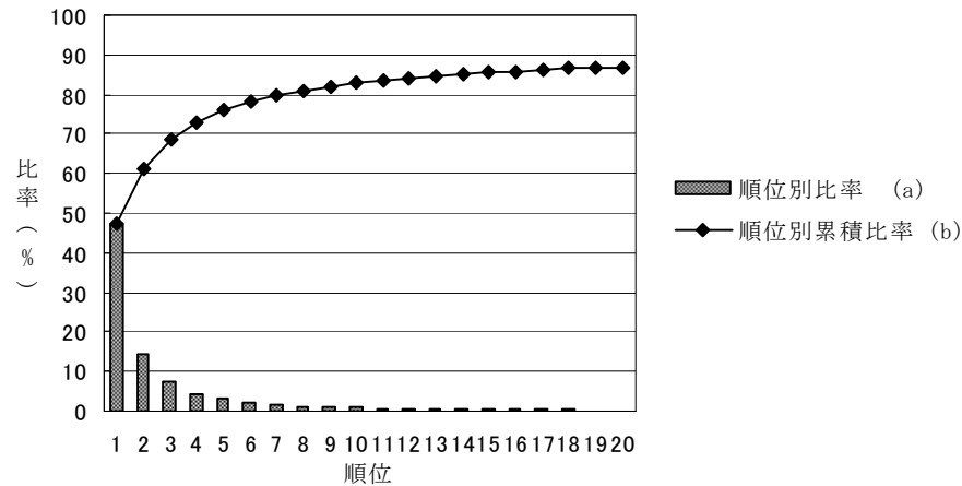
図2 [名詞+格助詞+動詞]型表現の GoogleN グラムにおける動詞の出現頻度順位別の動詞採録率(a)と順位別の動詞採録累積比率(b) (格助詞「を」、「が」、「に」に限定)
