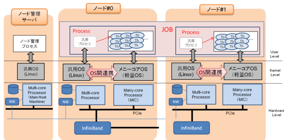
図1 メニーコア混在型並列計算機アーキテクチャとプロセスモデル
