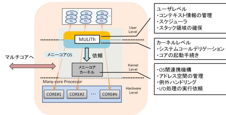
図 2 MULiTh とメニーコアカーネルの機能分担
