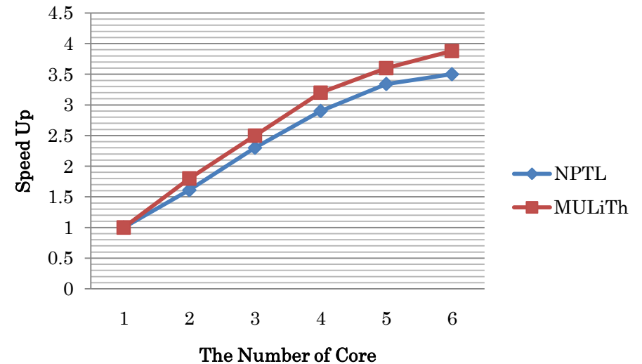
図 6 ベンチマーク実行時間の性能向上率
