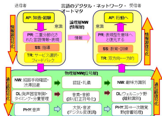
図3 ネットワークのOSI参照モデルに準拠した言語情報システム
