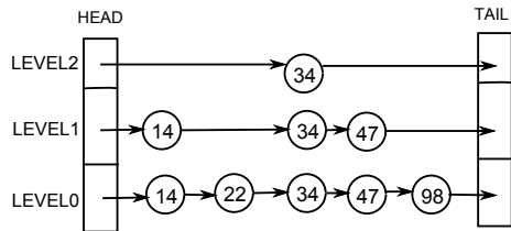
図 5 Skip list
