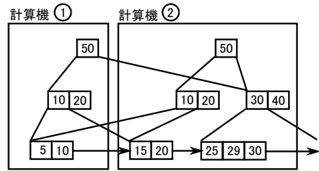
図 4 Fat-Btree の具体例
