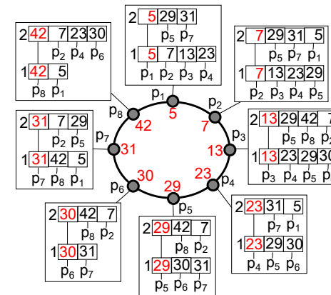
図 1 P-tree
