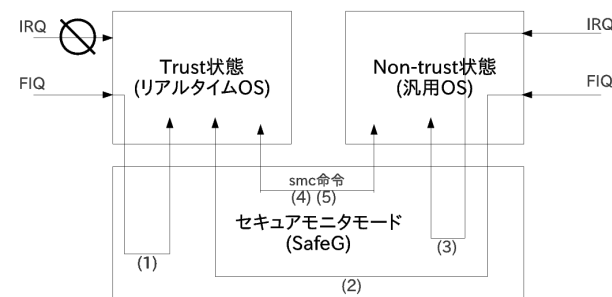
図 2 SafeG の実行パス Fig.2 Execution path of SafeG
