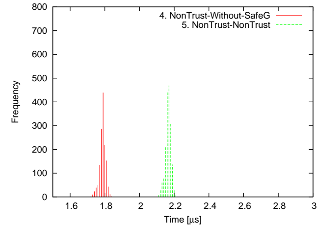
図 7 ノントラスト側 FMP の act.tsk 計測結果 Fig. 7 Evaluation results of API(act.tsk) on Non-trust side FMP
