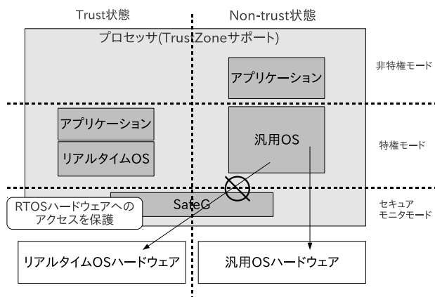
図 1 SafeG による方式 Fig.1 Concept of SafeG
