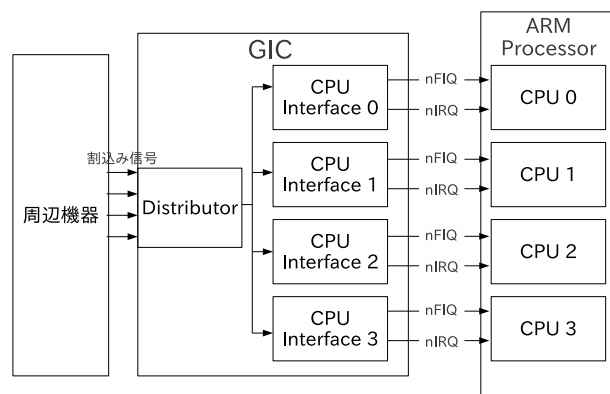
図 3 TrustZone 対応マルチコアプロセッサにおける割り込みアーキテクチャ Fig. 3 Interrupt Architecture for Multicore Processor with TrustZone
