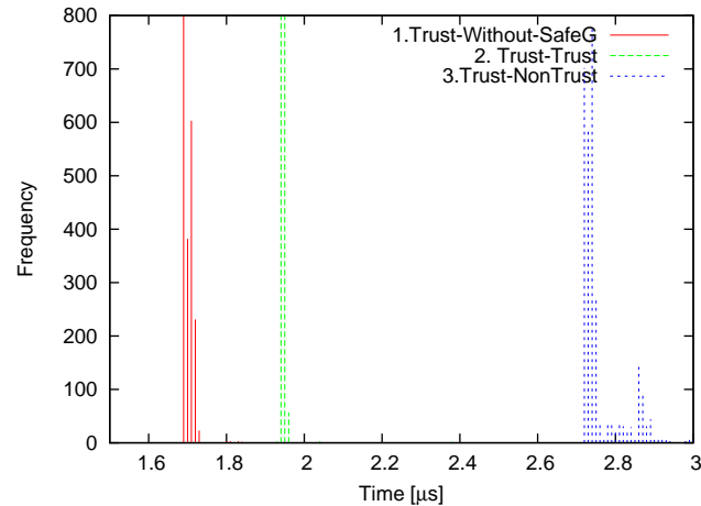
図 6 トラスト側 FMP の act.tsk 計測結果 Fig. 6 Evaluation results of API(act.tsk) on Trust side FMP
