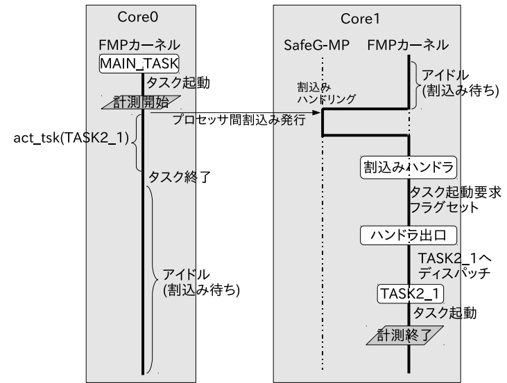
図 5 act_tsk 評価実験の内容
