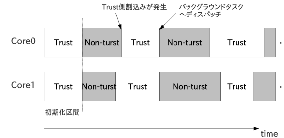
図 4 アイドルスケジューリング Fig.4 Idle scheduling
