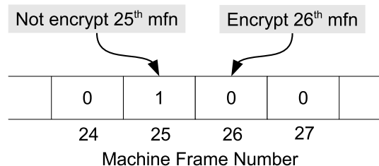
図 2 非暗号ページを表わすビットマップ
