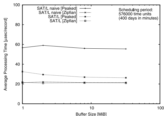
図 8 異なる書き込みバッファ管理方式に対するレコード処理時間の変化
