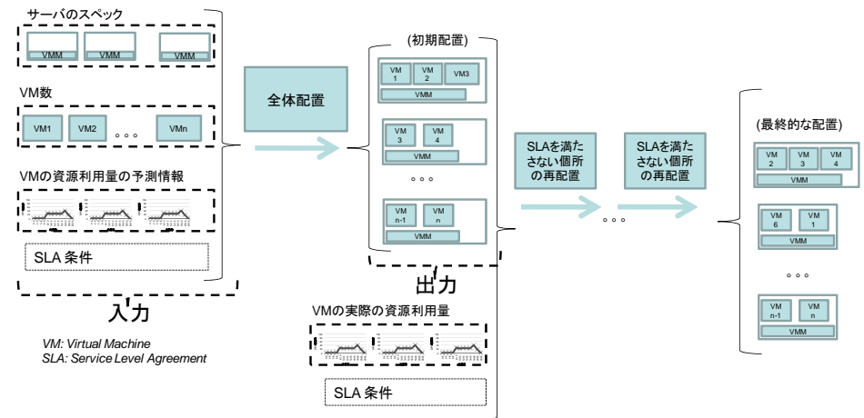
図 3 仮想マシン配置アルゴリズムの概要
