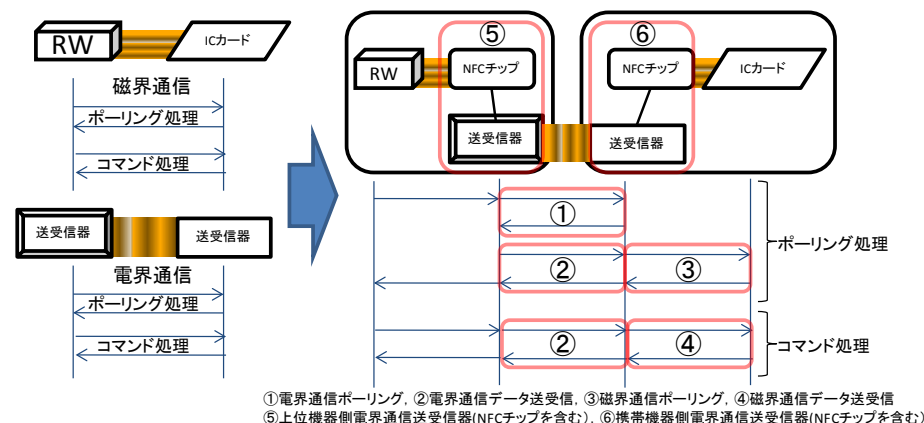
図 3 電界通信を追加することで生じる通信遅延箇所
