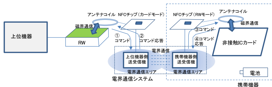
図 2 提案する構成方法
