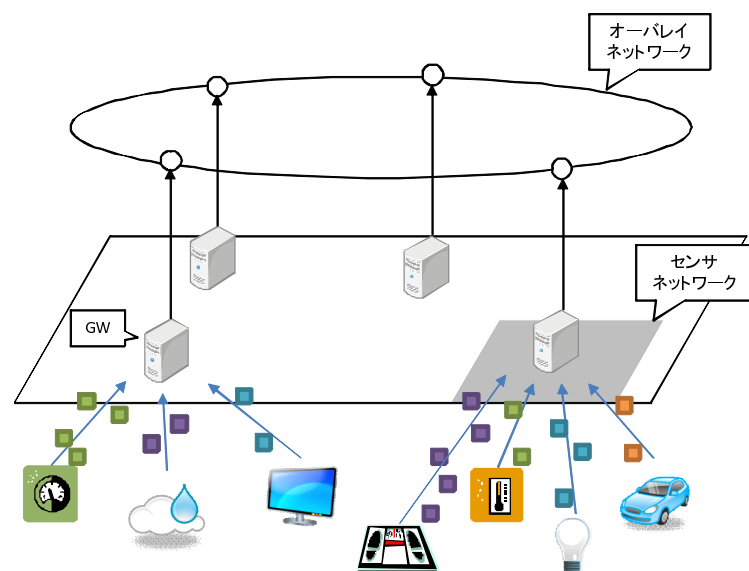
図 1 センサデータ収集システムの分散アーキテクチャ
