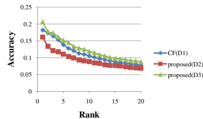
図 16 観測期間の長さに関する性能比較 Fig. 16 Performance comparison for the length of an observation period.
