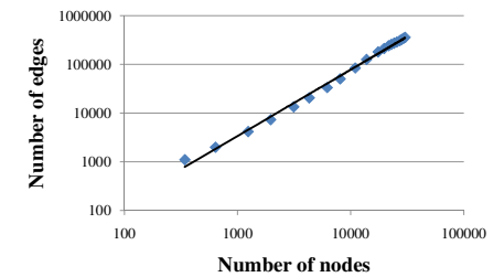
図 3 ノード数 n(t) に対するリンク数 e(t) (log-log scales) Fig. 3 Number of edges e(t) versus number of nodes n(t) in log-log scales.
