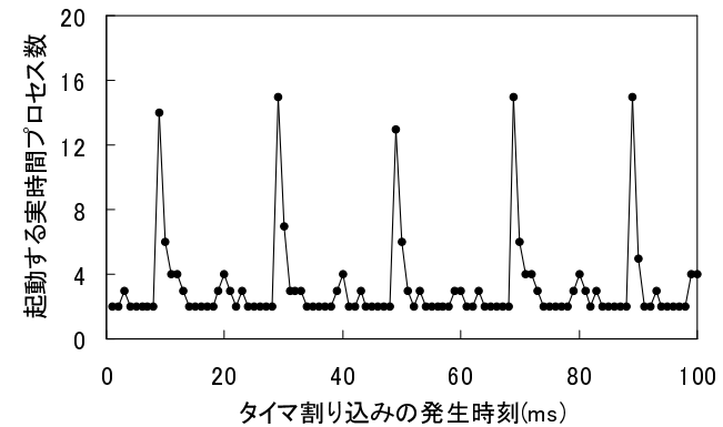
図 5 タイマ割り込みの発生時刻毎の起動する実時間プロセス数 (ART-Linux)
