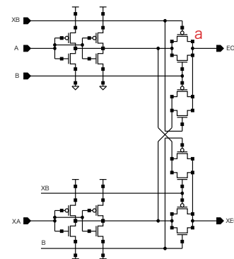
図1 LEORの回路図
