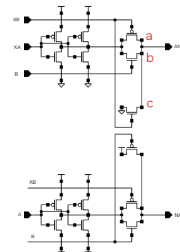
図2 LNORANDの回路図
