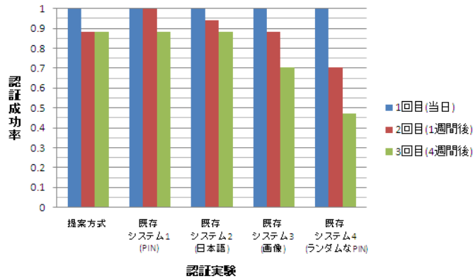
図 8 認証成功率
