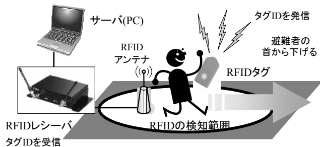
図 15 アクティブ RFID システムによるデータ取得方法 Fig. 15 Acquisition method of pedestrian data with the active RFID system
