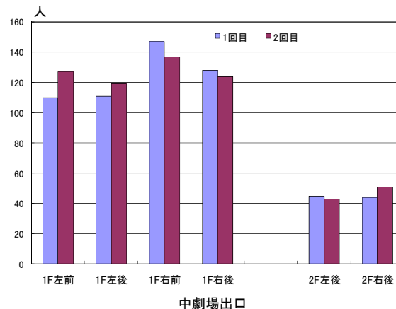
図 13 USV を用いたデータの取得結果 (劇場出口を通過した訓練参加者数の比較) Fig. 13 The number of evacuees passing through the exit
