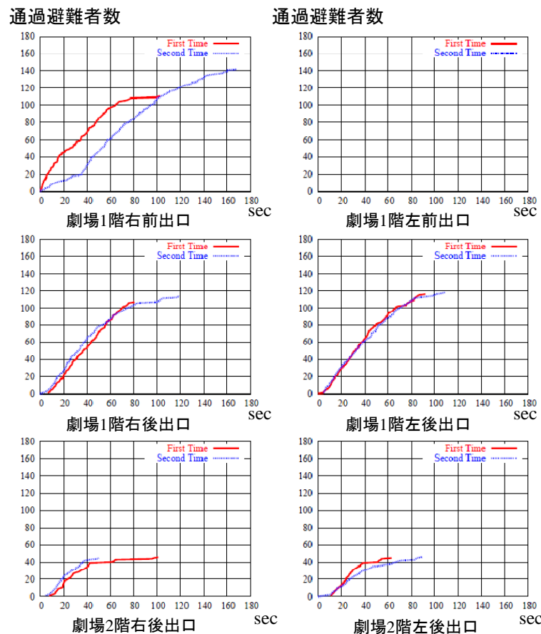
図 12 USV を用いたデータの取得結果 (劇場出口を通過した訓練参加者数の時間変化) Fig. 12 Time series of the number of evacuees passing through the exit
