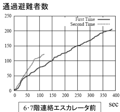
図 14 USV を用いたデータの取得結果 (6・7 階連絡エスカレータ前を通過する訓練参加者数) Fig. 14 Time series of the number of evacuees passing through the escalator from 7F to 6F
