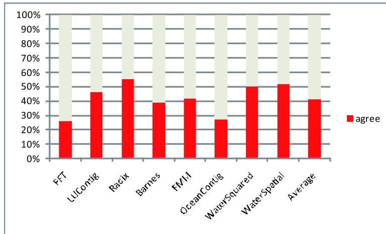
図 3 連想度=8, L1=32kB, L2=256kB での agree
