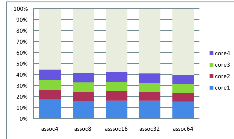
図 8 L1=32kB, L2=256kB でのコア局所性の連想度による変化
