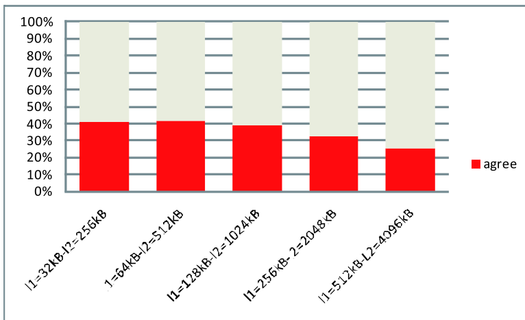
図 7 連想度=8 での agree の L1,L2 キャッシュ容量による変化
