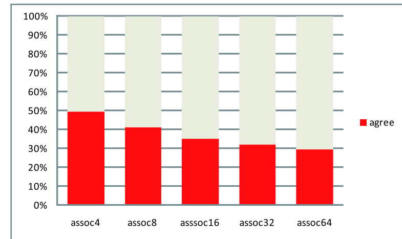
図 9 L1=32kB, L2=256kB での agree の連想度による変化
