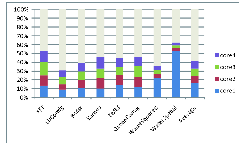
図 2 連想度=8,L1=32kB,L2=256kB でのコア局所性 Fig. 2 Access locality of cores when associativity=8, L1=32kB,L2=256kB.
