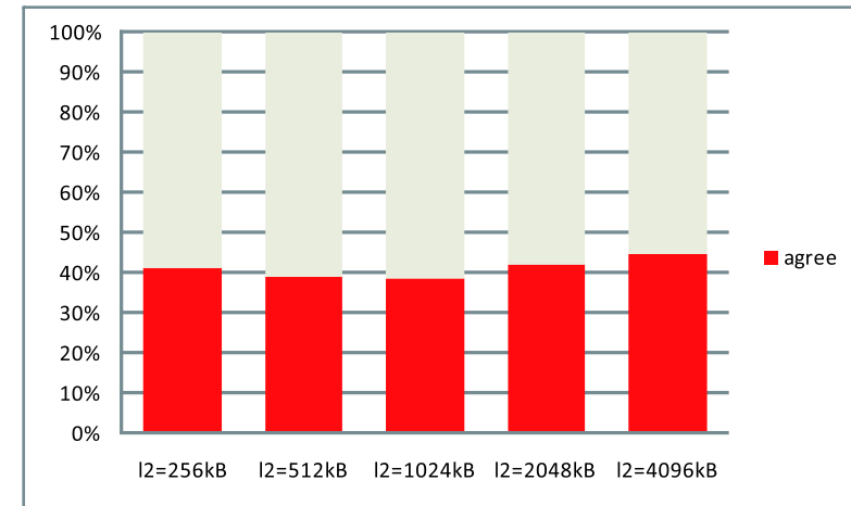
図 5 連想度=8, L1=32kB での agree の L2 キャッシュ容量による変化
