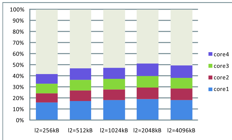
図 4 連想度=8, L1=32kB でのコア局所性の L2 キャッシュ容量による変化
