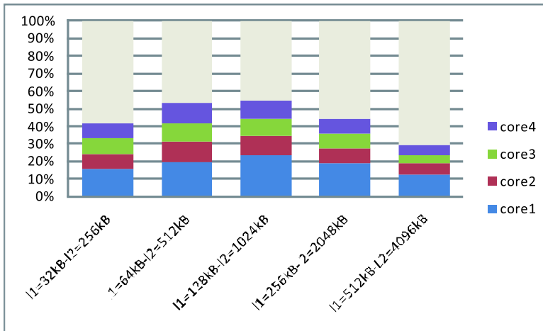
図 6 連想度=8 でのコア局所性の L1,L2 キャッシュ容量による変化
