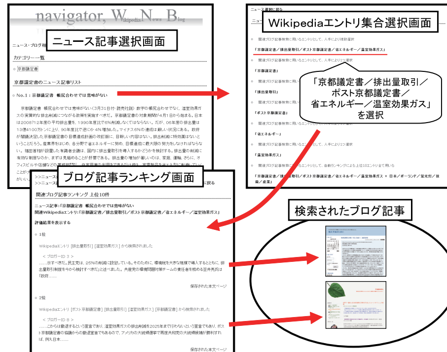
図 2 Wikipedia・ニュース・ブログ間の相補的ナビゲーションのためのインタフェース
